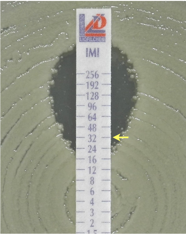
Example 3: A. baumannii , IMI MIC = 32 µg/mL
